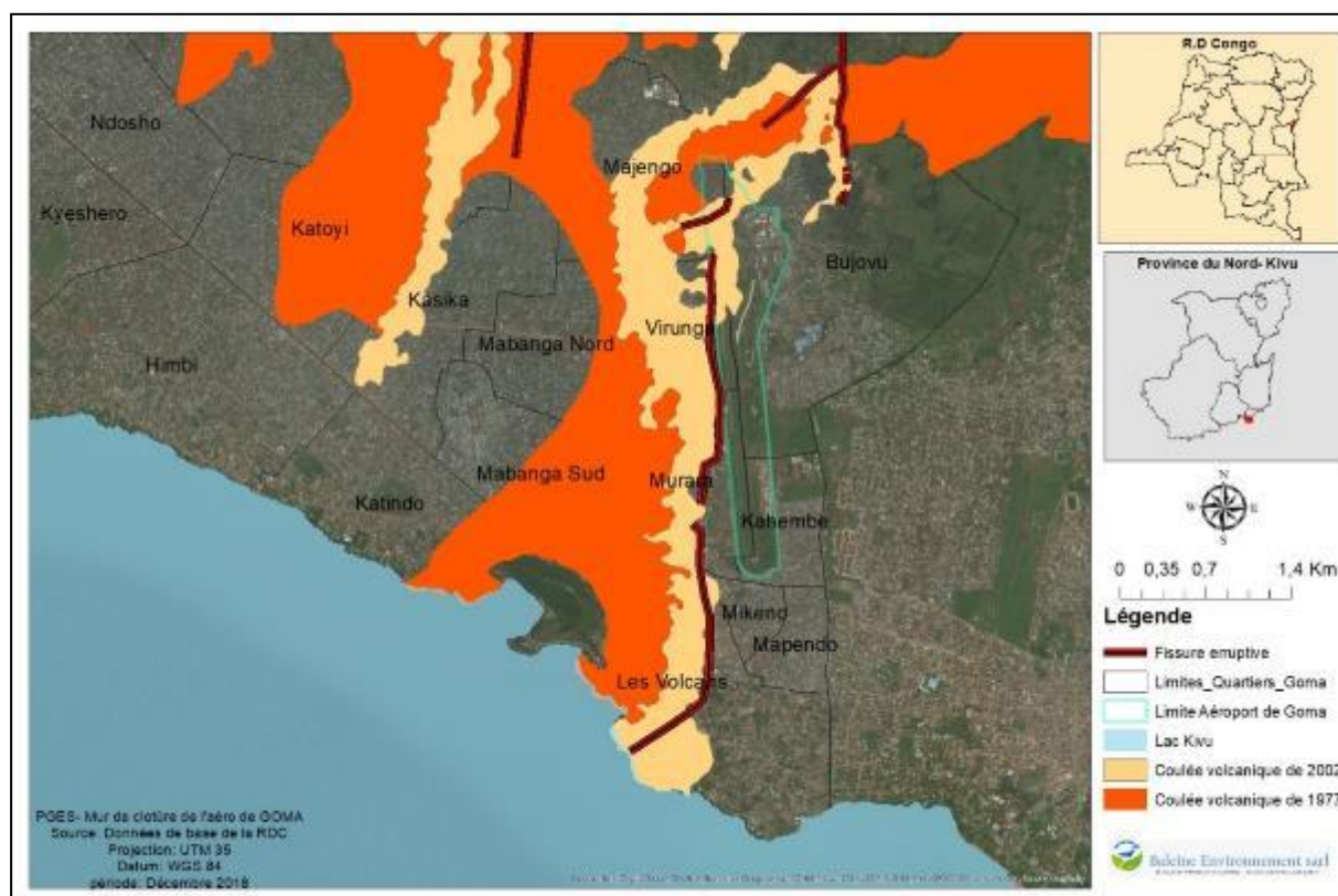
Carte 3 : Risques volcaniques et sismiques liés au projet (destinées de Base de la RDC projection UTM décembre 2018)
