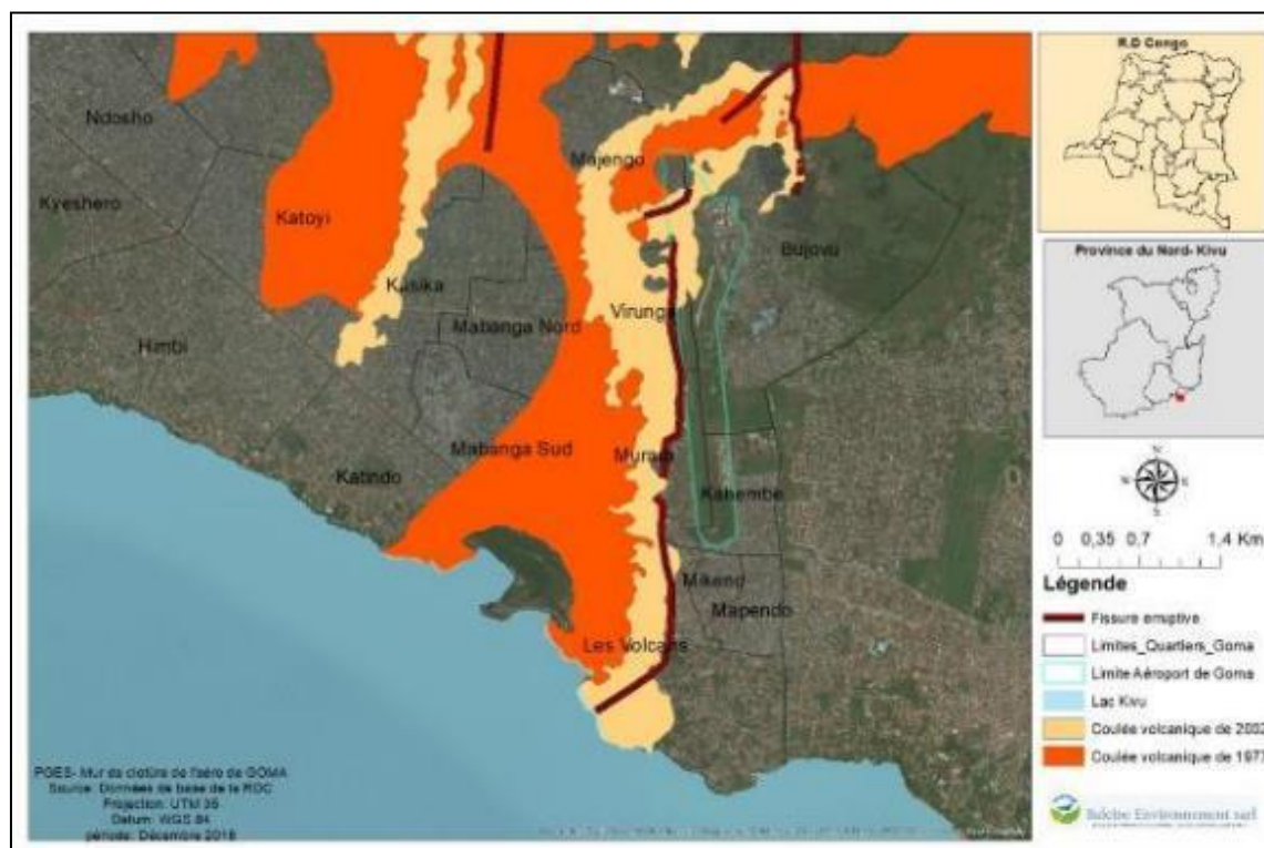
Carte 3 : Risques volcaniques et sismiques liés au projet
